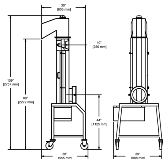
O MODELO COM ALIMENTAÇÃO DIRETA SE ACOPLA AO MOEDOR
