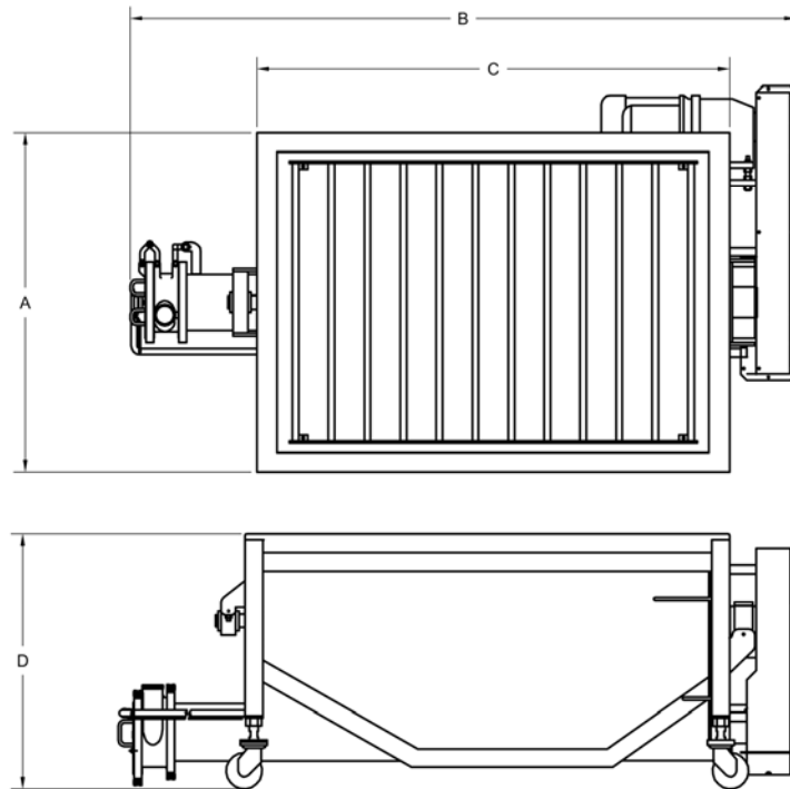
COCLEA PER TRASPORTO ORIZZONTALE
